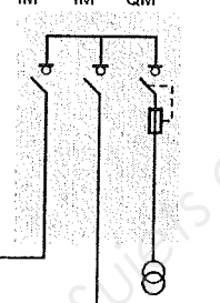
Poste de livraison HTA (abonnés à comptage)
