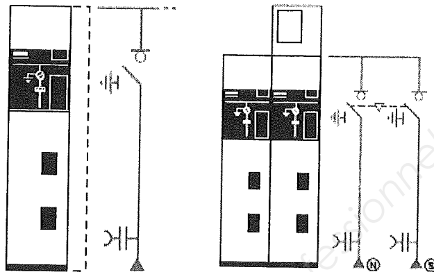
Alimentation câbles pour arrivée prioritaire et secours NSM-câbles (750 mm)
