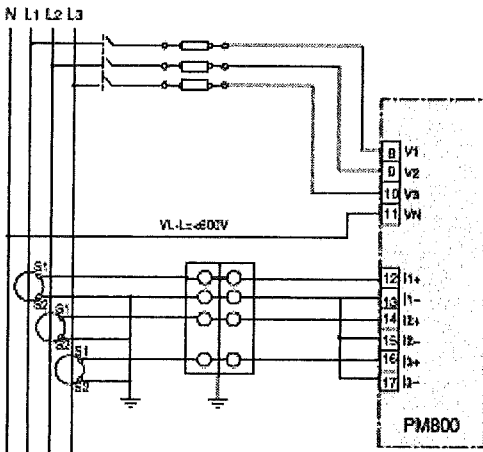
Figure 4-6 : Raccordement triphasé en étoile en 4 fils, avec raccordement direct de la tension et 3 TC
