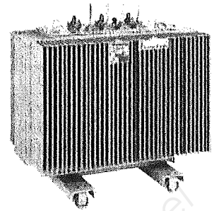
1000 kVA - 20 kV / 400 V
