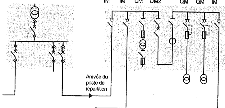
Poste mixte DP/Abonnés
