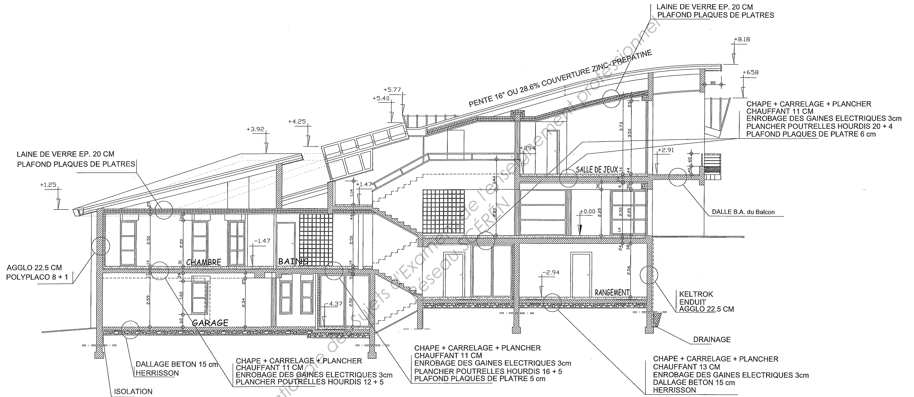
COUPE AA
