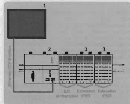
Entrées/Sorties locales
