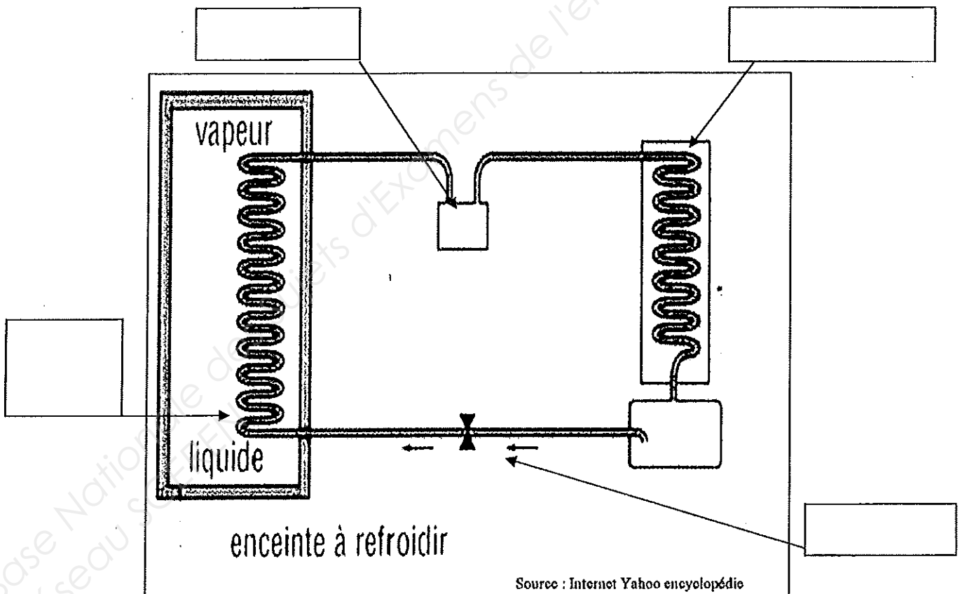
Schéma de principe d'un appareil producteur de froid
