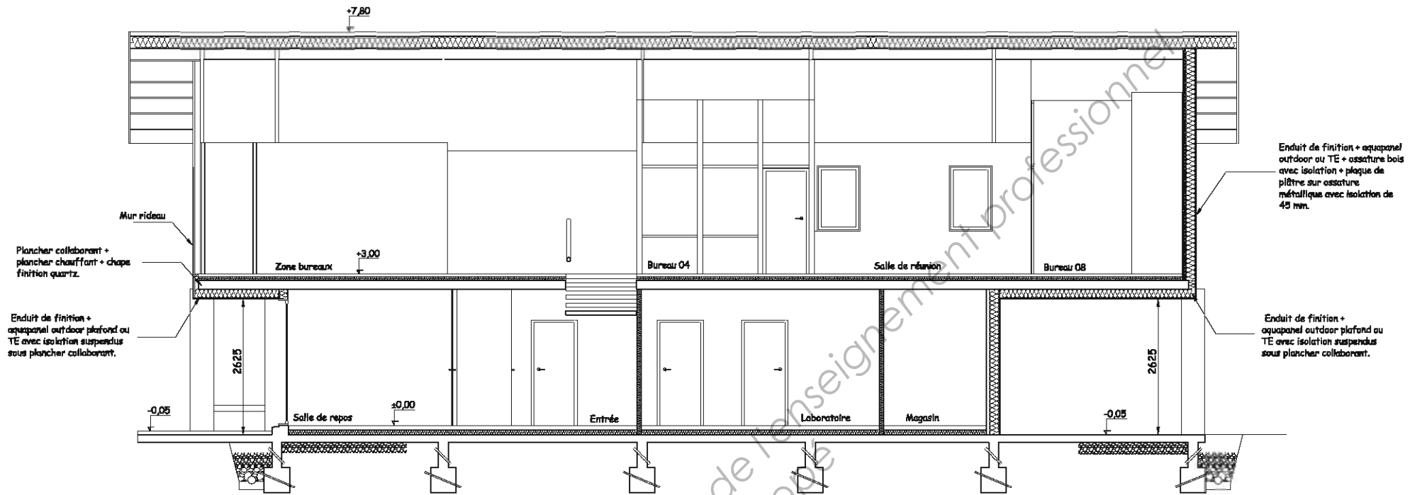
COUPE BB Echelle : 1/75
