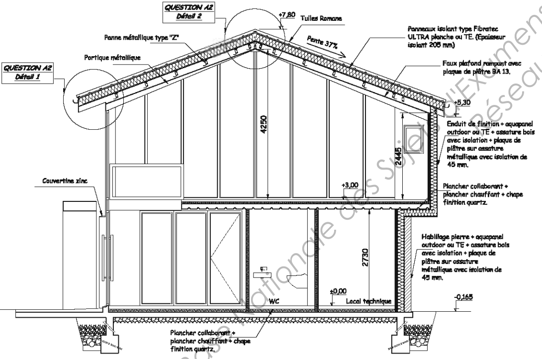
COUPE AA Echelle : 1/75
