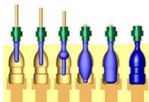
Processus d'étirage-soufflage d'une préforme. (Extrait de Wikipedia)
