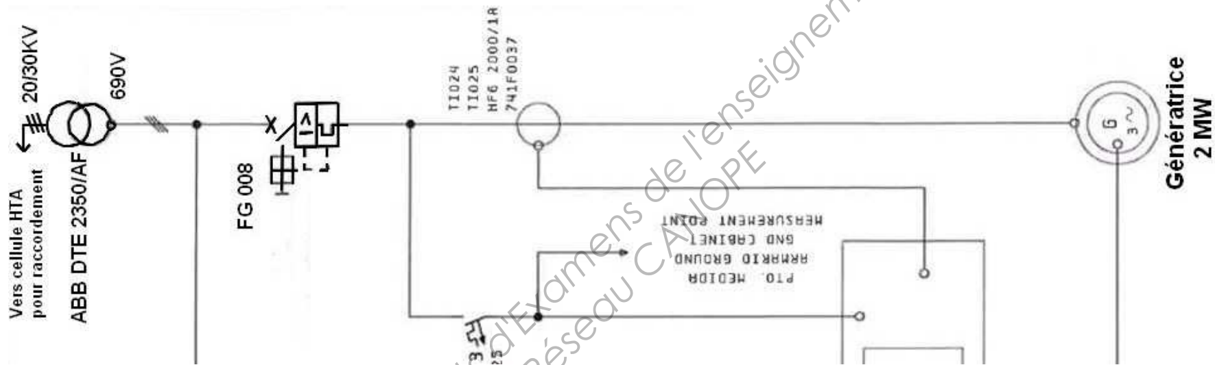
Schéma partiel de raccordement de l'éolienne N°6
