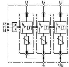
Schéma de principe du circuit DG M TNC FM
