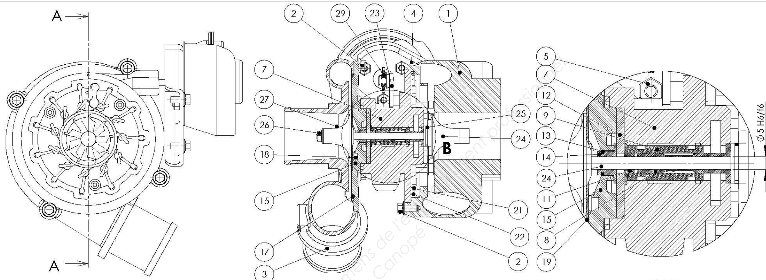
COUPE A-A ECHELLE 2 : 3
