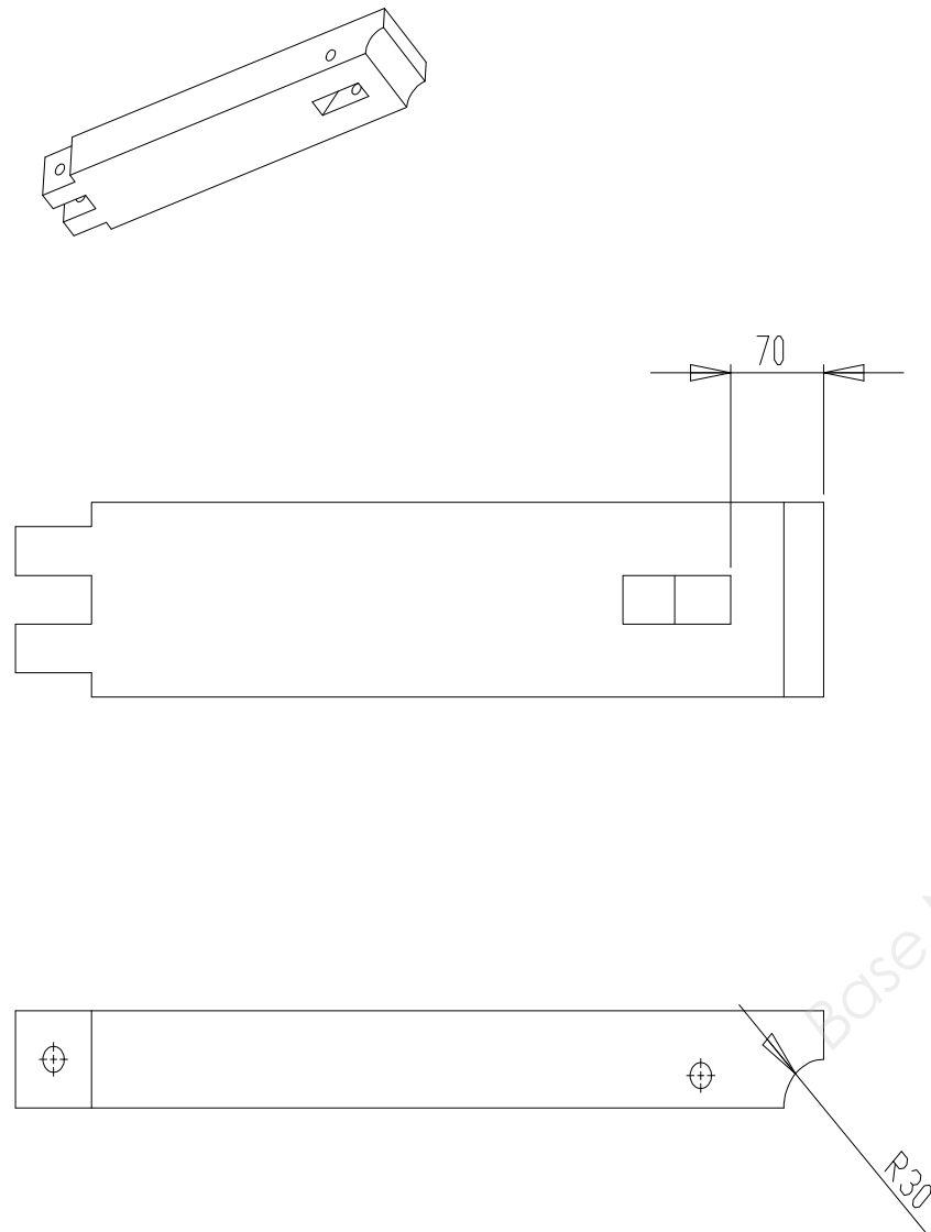
TRAVERSE DE POTENCE Repère : 3
