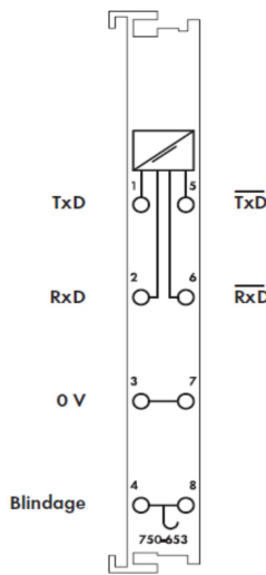
Illustration : série 750 / représentation voir page 24 / Livraison sans Mini-WSB, repérage série 750 / 753, voir pages 10 ... 11 / 12 ... 13
