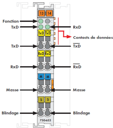
Illustration : série 750 / représentation voir page 24 / Livraison sans Mini-WSB, repérage série 750 / 753, voir pages 10 ... 11 / 12 ... 13
