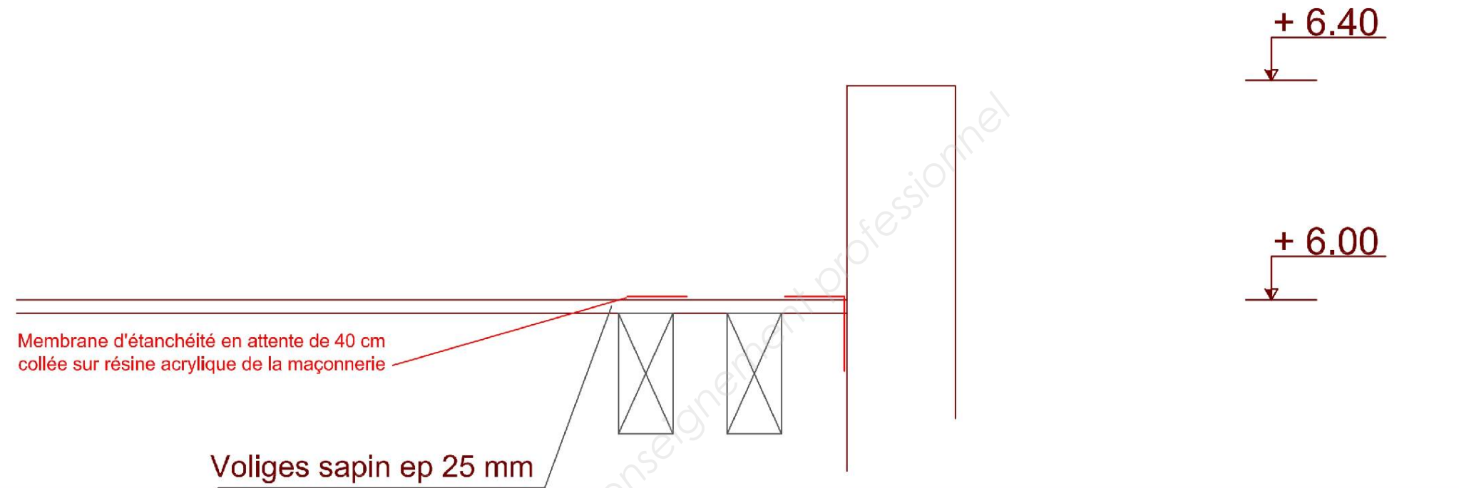
Détail n°1 - Echelle 1/10
