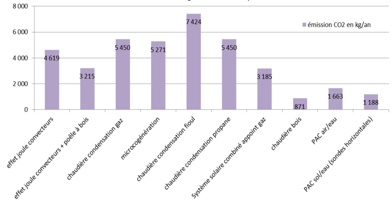
Emission de CO 2 annuelle liée à la consommation d'énergie pour le chauffage d'une maison existante de 120 m 2 construite entre 1975 et 1981 en zone climatique H1 (Trappes) - avec des besoins de chauffage de 20 000 kWh/an
