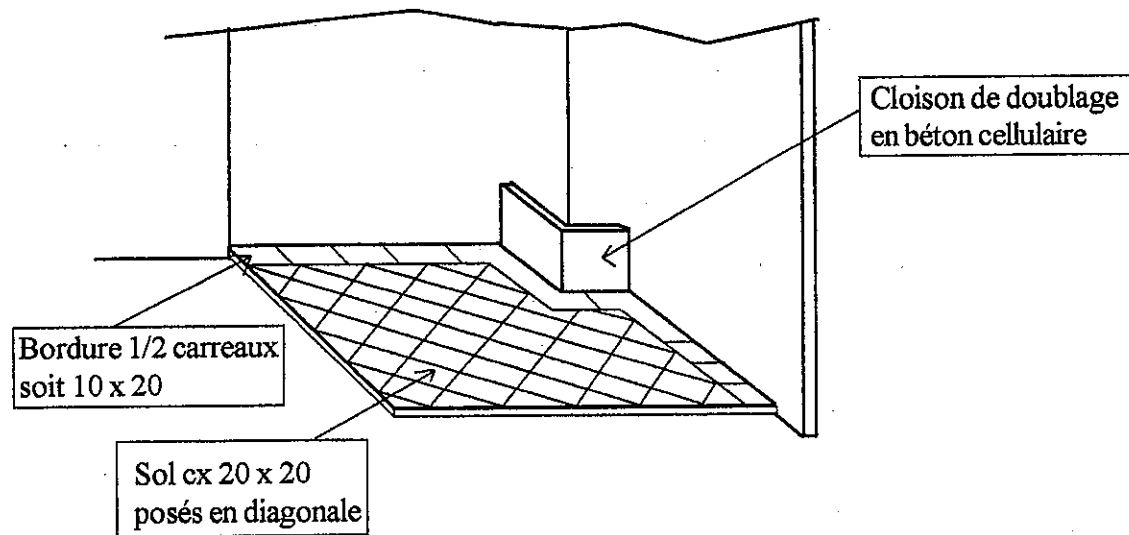
Aspect de l'ouvrage à réaliser
