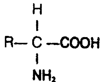
Molécule 4
