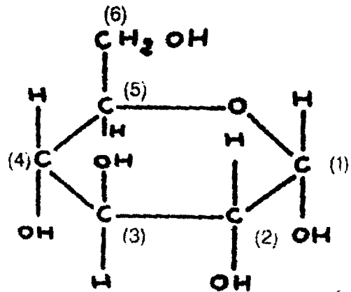
Molécule 3
