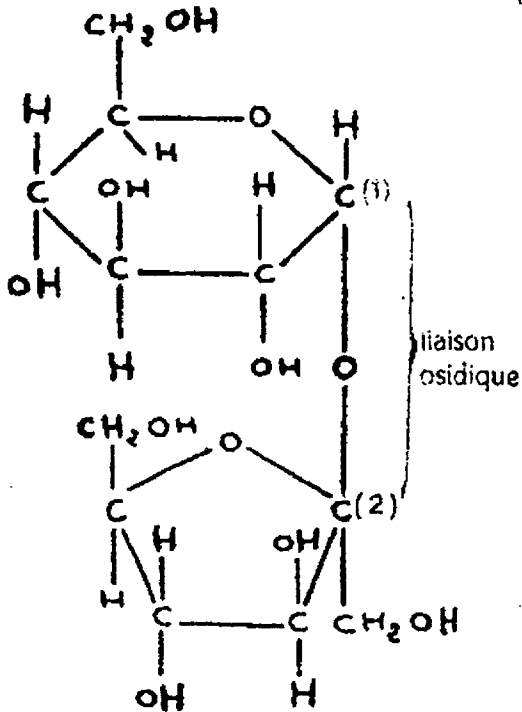
Molécule 2
