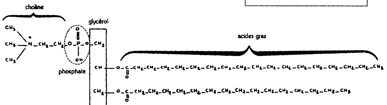
Molécule 5
