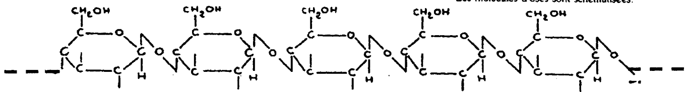
Molécule 1
