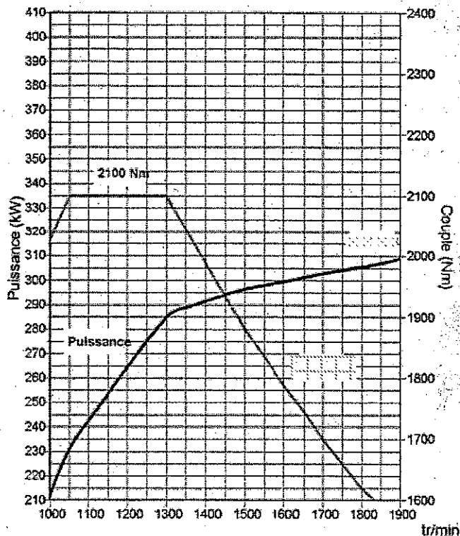
Courbes de performances du moteur DC 1214
