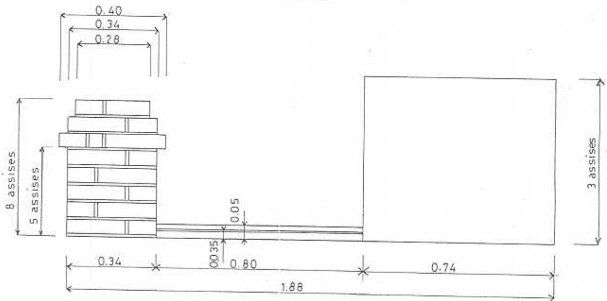
ELEVATION
