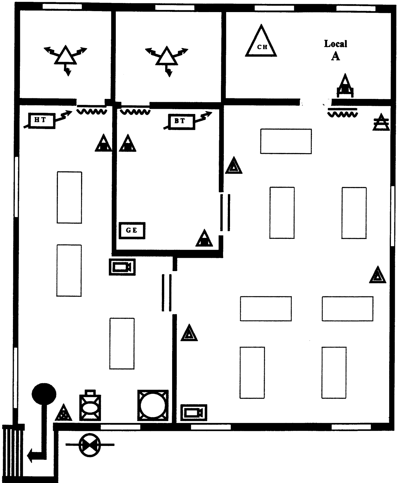
Plan du rez-de-chaussée. Laverie
