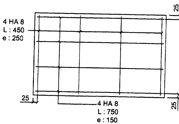
Armature de la dalle préfabriquée
